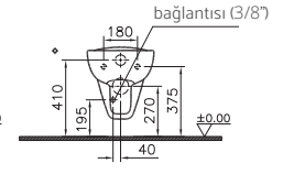
Sıva altı bağlantı
