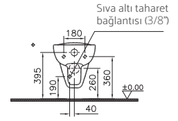
Sıva altı bağlantı
