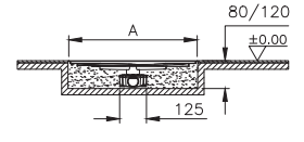
Yandan Çıkışlı Sifon Kesit
