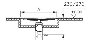
Altan Çıkışlı Sifon Kesit
